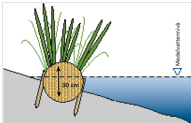
Figur 1: Vegetationen är beroende av kontinuerlig vattentillgång och strandrullen ska monteras på rätt nivå i förhållande till medelvattennivån.
